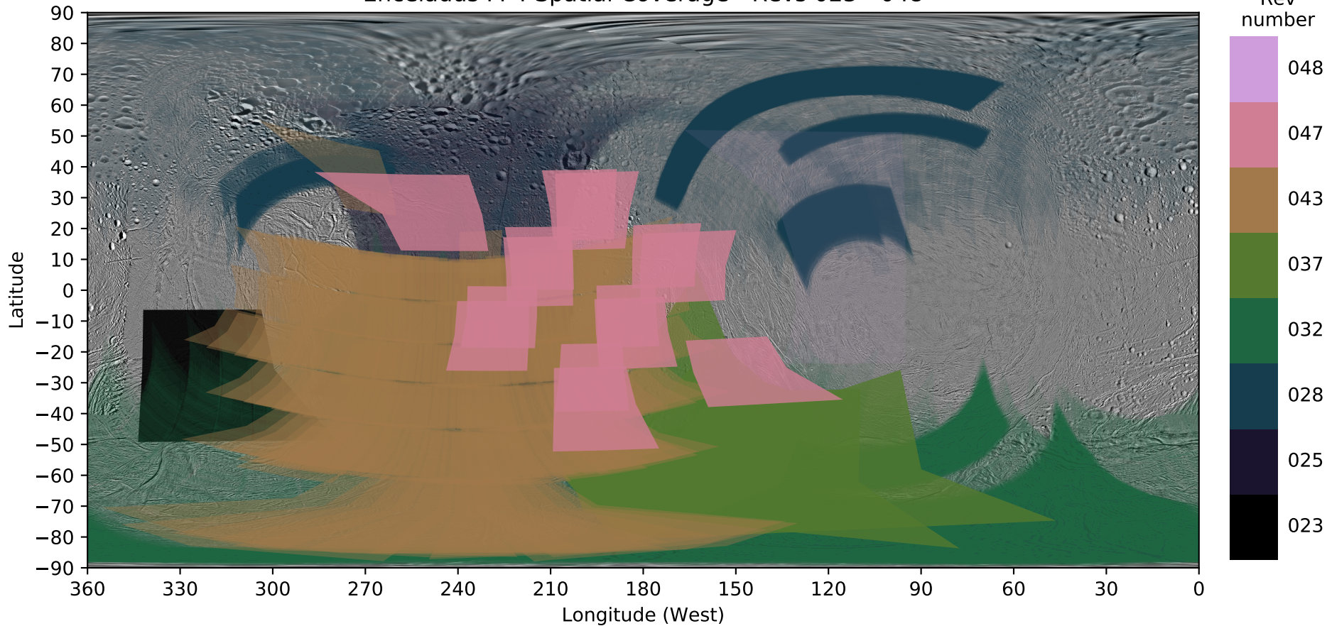
Enceladus FP4 Spatial Coverage - Revs 023 - 048
