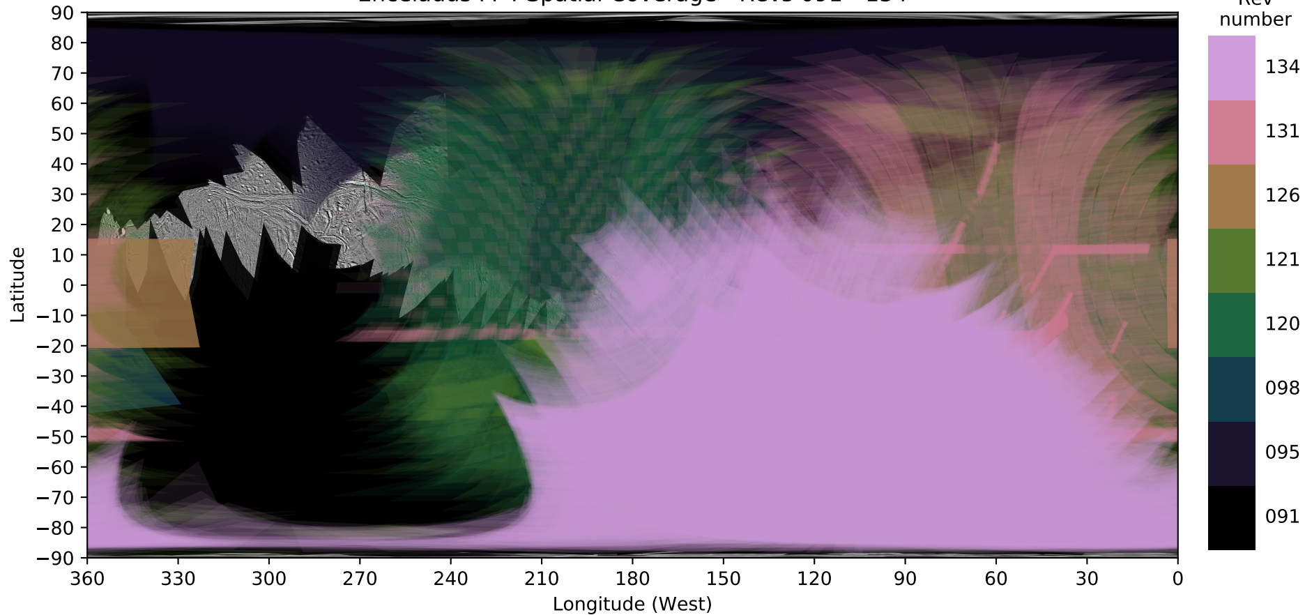
Enceladus FP4 Spatial Coverage - Revs 091 - 134
